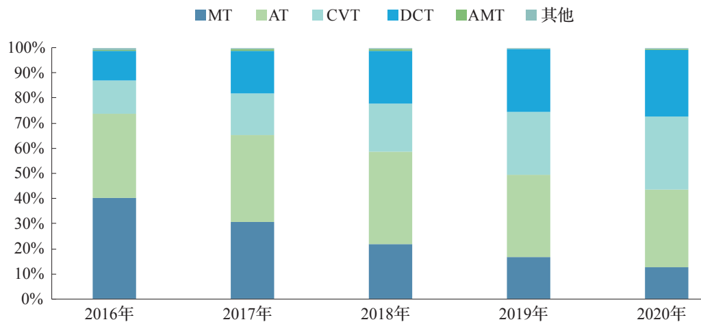
图 28 乘用车变速器技术搭载率
